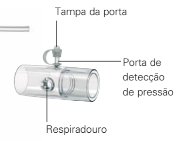
Conector de porta de expiração em linha
